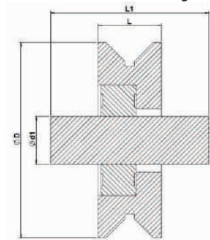
IMAGEM 06 – DESENHO TÉCNICO ROLDANAS DE AÇO PERFIL – V COM ROLAMENTO E PINO.
