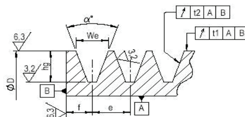
DIMENSÃO TIPO DE PERFIL DO CANAL Z A B C D SPZ SPA SPB SPC 3V 5V 8V We 9,7 12,7 16,3 22 32 9,7 12,7 16,3 22 8,9 15,2 25,4 f (Polia Ferro) 9,85 11,35 13,15 17 23 9,5 11,35 13,15 17 9,45 13,6 19,7 f (Polia Alumínio) 8,35 9,85 11,65 - - 8,35 9,85 11,65 - - - - e 12 15 19 25,5 37 12 15 19 25,5 10,3 17,5 28,6 hg 9 13,8 17,5 19,5 28 11 13,8 17,5 23,8 9 15,2 25,4 a ±0,5° 34° D£80 D£118 D£190 D£315 ---- D£80 D£118 D£190 D£315 ---- ---- ---- 36° ---- ---- ---- ---- D£475 ---- ---- ---- ---- D £ 90 ---- ---- 38° D>80 D>118 D>190 D>315 D>475 D>80 D>118 D>190 D>315 90< D£150 D £ 250 D £ 400 40° ---- ---- ---- ---- ---- ---- ---- ---- ---- 150< D£300 250< D£ 400 400< D£ 560 42° ---- ---- ---- ---- ---- ---- ---- ---- ---- D > 300 D > 400 D > 560 Tolerância em e ± 0,3 ± 0,3 ± 0,4 ± 0,5 ± 0,6 ± 0,3 ± 0,3 ± 0,4 ± 0,5 ± 0,25 ± 0,25 ± 0,4 Soma dos desvios de e ± 0,6 ± 0,6 ± 0,8 ± 1 ± 1,2 ± 0,6 ± 0,6 ± 0,8 ± 1 ± 0,5 ± 0,5 ± 0,8 Ø D mín. Recomendado 50 75 125 200 355 63 90 140 224 67 180 315
