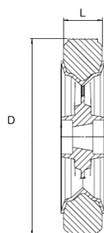
Fig.17 - Dimensões do aro de 8" bipartido com pneu
