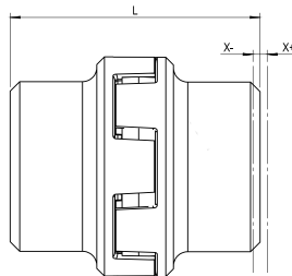
Desalinhamento axial
